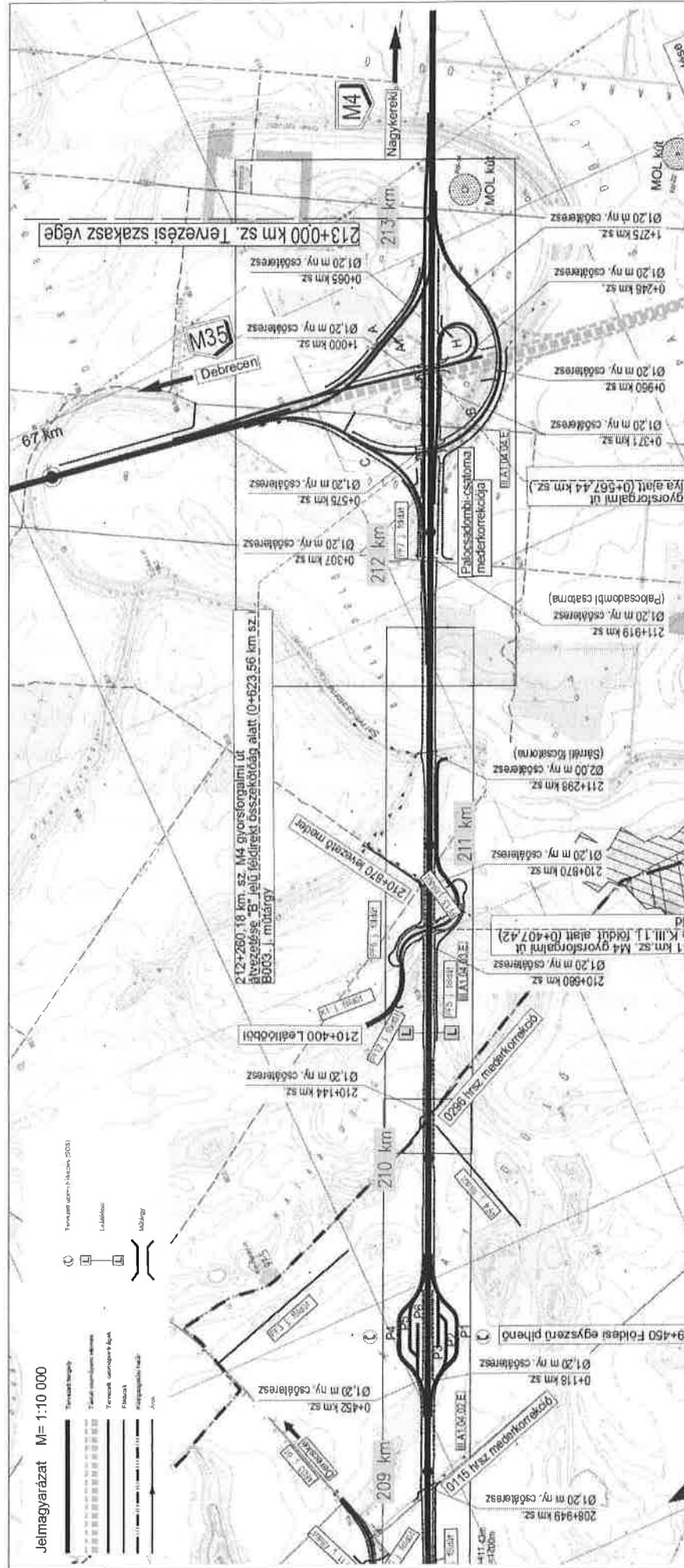
Átnézeti tervlap az M4 nyomvonalal (1. tervezési terület)
