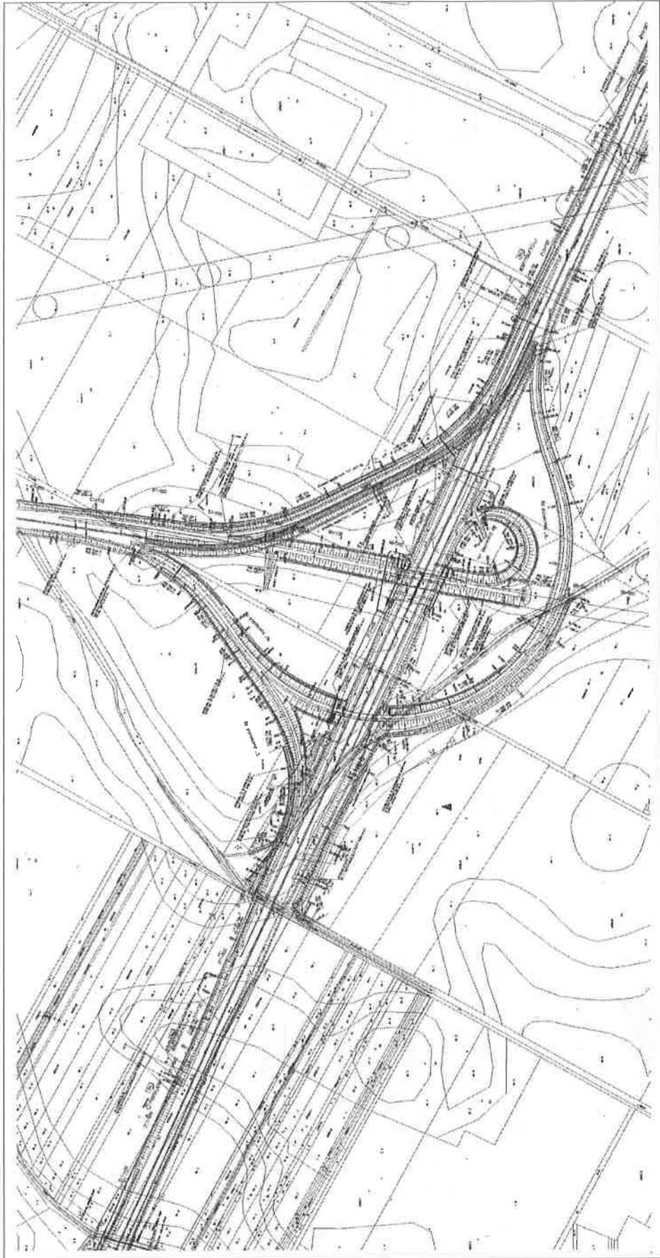
Derecske csomópont tervezett átépítése (1. tervezési terület)
