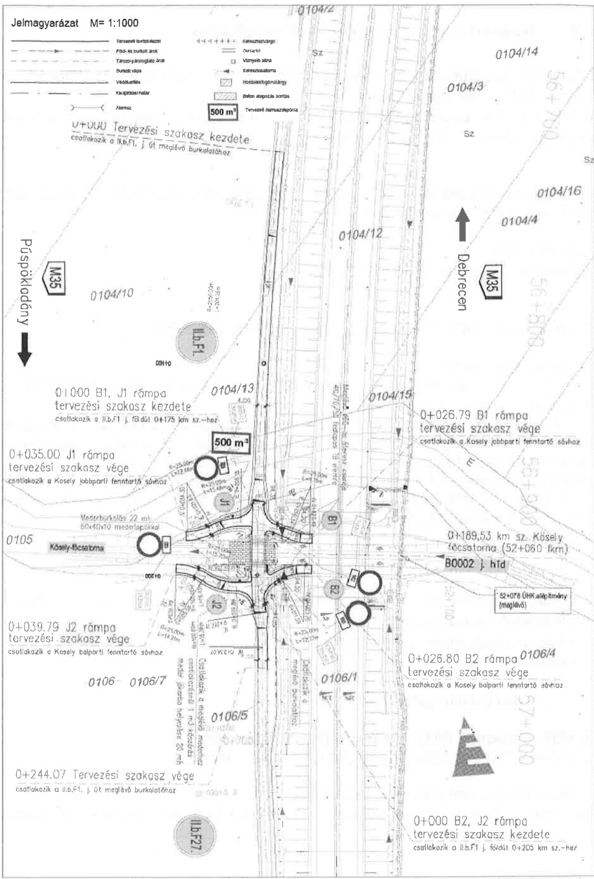
Útépítési terv (2. tervezési terület)
